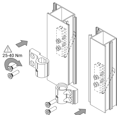
FIXATION TRADITIONNELLE AVEC CONTRES-PLAQUES FIXAÇÃO TRADICIONAL COM CONTRA CHAPADOS
